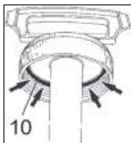
Fig. 10: Om de tank goed af te sluiten moet de deksel dichting (10) altijd goed met siliconenvet ingesmeerd zijn.
